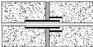
Rohrdurchführung
