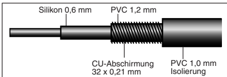
Heizleitung NH2GYQUY 90 (DSVG)
